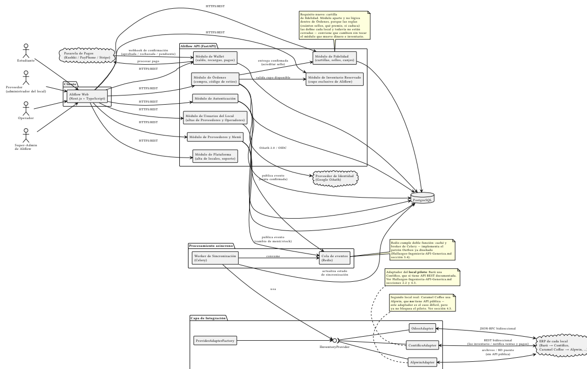
Figura 5: Diagrama de componentes de Aliflow
