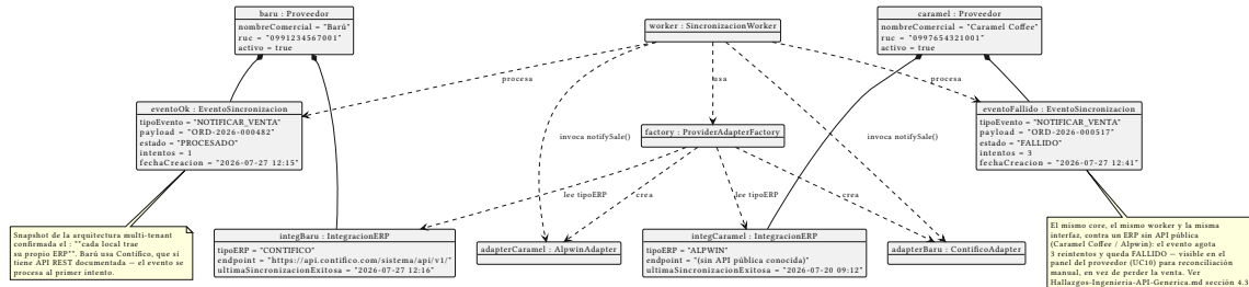
Figura 4: Diagrama de objetos: integración ERP
