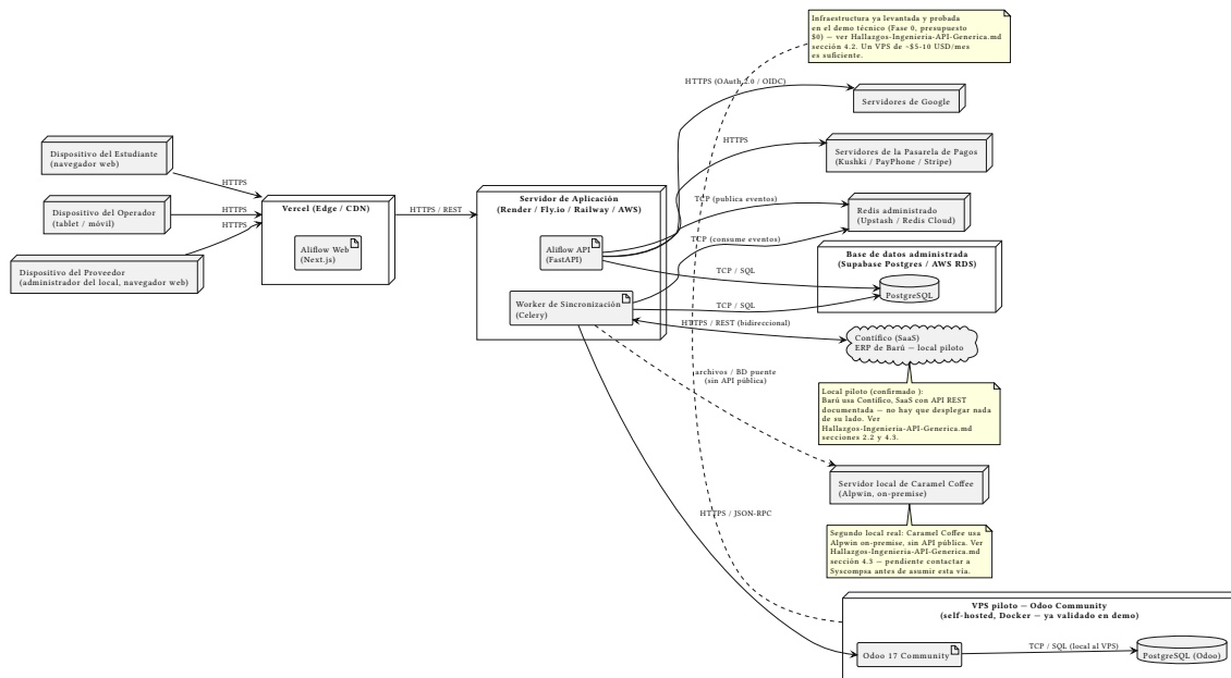
Figura 6: Diagrama de despliegue de Aliflow
